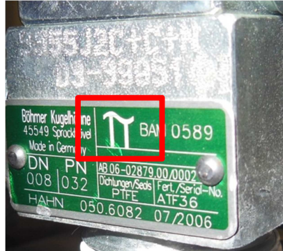
Kugelhahn mit \pi -Zeichen
