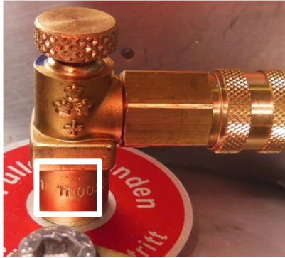
Schnüffelventil mit \pi -Zeichen
