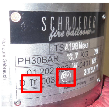
Gasbehälter mit \pi - und TÜV-Zeichen
